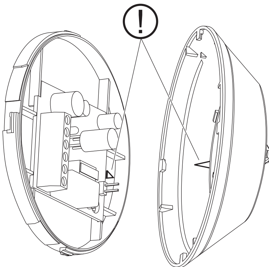
3. ÁBRA. Fedél és hátlap jelzéseinek összeigazítás az érzékelő házának visszazárásakor.
